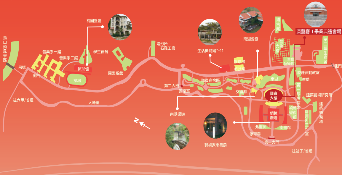
校園配置圖
